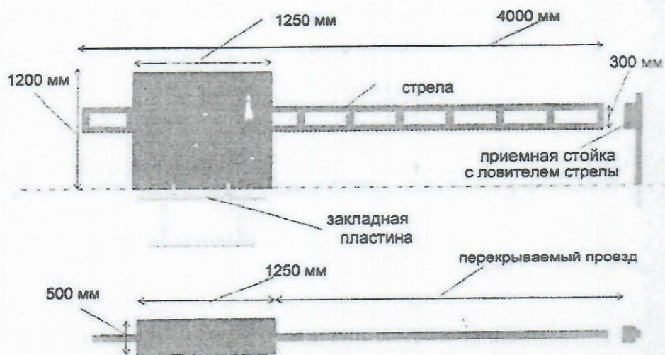
Рис. 2. Габаритные размеры
