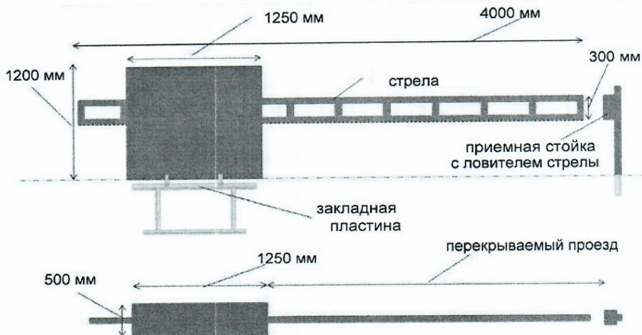
Рис. 2. Габаритные размеры
