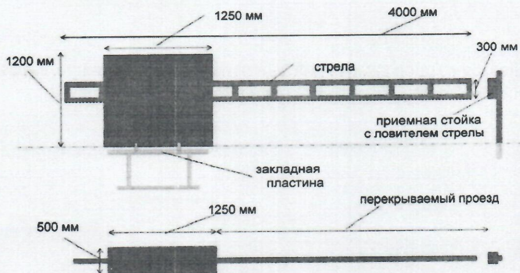
Рис. 2. Габаритные размеры
